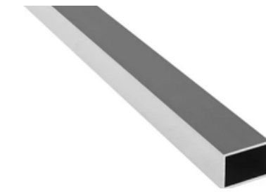
Profil 30x20x2mm
